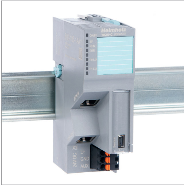
EtherCAT
