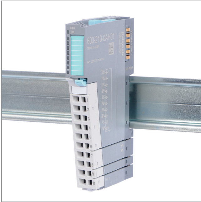
DI 8 x 24 VDC
