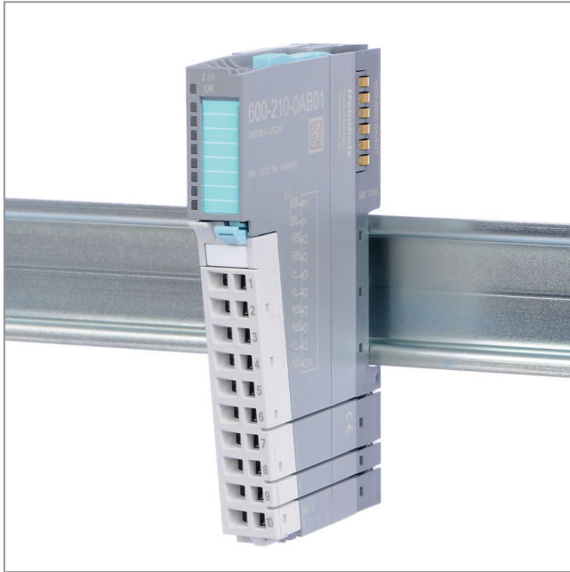
DI 2 x 24 VDC
